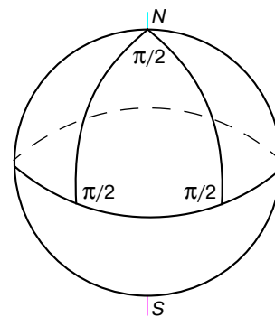
Рис. 1. Сферический треугольник.
