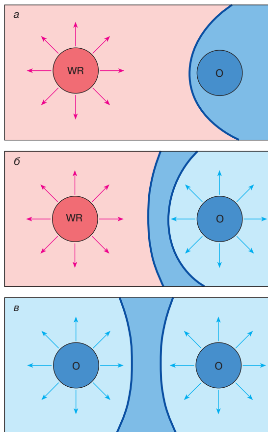
Рис. 1. Три вида взаимодействия звездных ветров в тесной двойной системе: а – (WR+O)-система. Звездный ветер звезды О пренебрежимо мал. Наблюдается ударная волна, образованная в результате столкновения сверхзвукового ветра звезды WR с поверхностью звезды О; б – (WR+O)-система. Столкновение двух звездных ветров, истекающих из звезды WR и звезды О. Наблюдается система из двух ударных волн, сформированных в ветре звезды WR и О-звезды. Эта система из двух ударных волн расположена ближе к О-звезде, поскольку поток кинетической энергии ветра О-звезды меньше, чем в случае звезды WR; в – (O+O)-система. Столкновение двух звездных ветров равной мощности. Формируется система из двух ударных волн, расположенная посередине между компонентами
