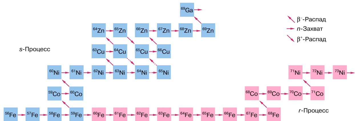
Рис. 3. Цепочки быстрого и медленного захвата нейтронов ( r - и s -процессы) для ядра ^{56}\text{Fe} . Точечные стрелками представлены альтернативные каналы образования ^{65}\text{Cu}
