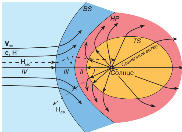
Рис. 2. Общая картина взаимодействия солнечного ветра с межзвездной средой. BS – головная ударная волна, HP – гелиопауза или граница Солнечной системы, TS – ударная волна в солнечном ветре, N_{MC} – атомы водорода, проникающие в солнечный ветер из межзвездной среды, N_{CB} – атомы водорода, возникшие после перезарядки N_{MC} на протонах солнечного ветра
