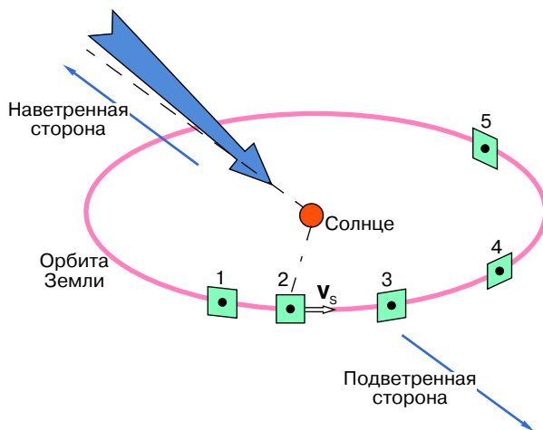
Рис. 3. Принципиальная схема измерений рассеянного солнечного излучения прибором, установленным на борту спутника Земли. Стрелка указывает направление движения атомов межзвездной среды, которые проникают в Солнечную систему. Белый квадрат указывает на плоскость, в которой вращается прибор, установленный для измерений, V_s – вектор скорости Земли, 1–5 – положения прибора в пяти сеансах
