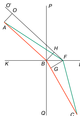
Рис. 1. Чертеж из работы Х. Гюйгенса “Трактат о свете”, поясняющий доказательство принципа Ферма на основании закона преломления
