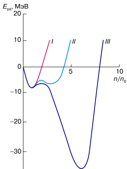
Рис. 1. Зависимость удельной энергии связи, взятой со знаком минус, от плотности ядерной материи. За единицу плотности ядерной материи принята нормальная ядерная плотность n_0
