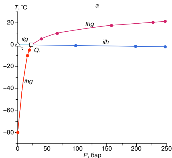
Рис. 7. P, T-фазовая диаграмма системы метан – вода; а – в интервале от 0 до 250 бар; б – в интервале от 0 до 15 кбар. Q_1 – четырехфазное невариантное равновесие ( ilh ), Q_h – четырехфазное невариантное равновесие ( lh_xg ), где i – лед, l – жидкая водная фаза, h и h_x – гидратные фазы КС-I и неизвестной структуры соответственно, g – газовая (флюидная) фаза (фазы расположены в порядке возрастания в них содержания метана); \tau – трехфазное невариантное равновесие ( ilg ) в унарной системе вода; \nabla – разложение гидрата h при P, T-условиях, где он метастабильен
