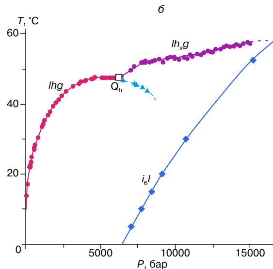
Рис. 7. P, T-фазовая диаграмма системы метан – вода; а – в интервале от 0 до 250 бар; б – в интервале от 0 до 15 кбар. Q_1 – четырехфазное невариантное равновесие ( ilh ), Q_h – четырехфазное невариантное равновесие ( lh_xg ), где i – лед, l – жидкая водная фаза, h и h_x – гидратные фазы КС-I и неизвестной структуры соответственно, g – газовая (флюидная) фаза (фазы расположены в порядке возрастания в них содержания метана); \tau – трехфазное невариантное равновесие ( ilg ) в унарной системе вода; \nabla – разложение гидрата h при P, T-условиях, где он метастабильен
