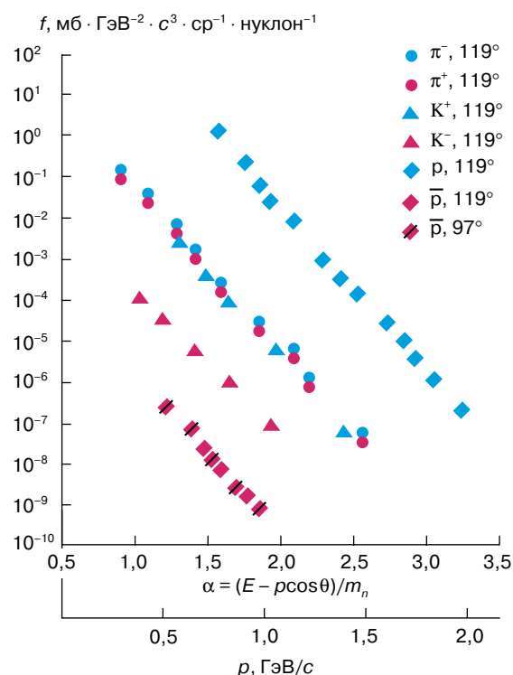
Рис. 2. Зависимость инвариантных функций различных кумулятивных частиц от их величин \alpha . Нижняя шкала абсцисс — импульс кумулятивных протонов при соответствующем \alpha .
