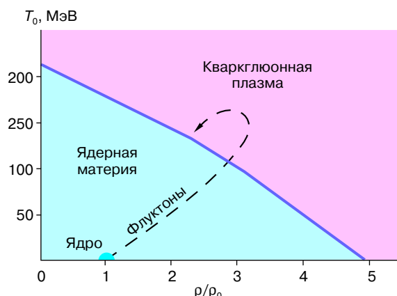
Рис. 5. Диаграмма фазового состояния вещества при различных температурах T и плотностях \rho/\rho_0 . Плотность дана относительно средней плотности ядра.
