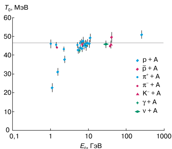
Рис. 3. Зависимость наклонов инвариантных функций кумулятивных протонов, вылетающих под углом 120^\circ , от энергии различных налетающих частиц.
