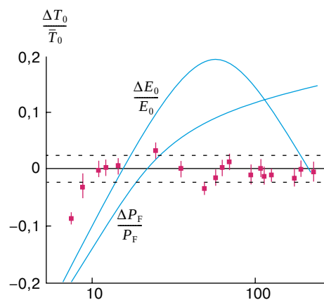
Рис. 4. Зависимость разности наклонов инвариантной функции кумулятивных протонов, нормированных на средний наклон, от массы ядра мишени. Кривые представляют относительные изменения энергии связи и фермиевского импульса для разных ядер-мишеней.
