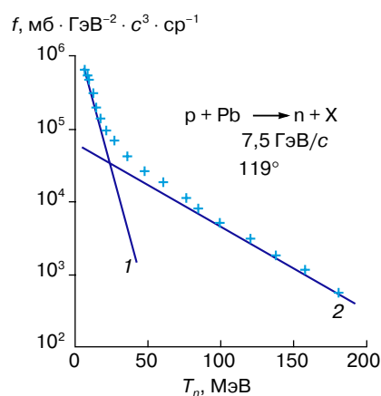
Рис. 1. Зависимость инвариантной функции кумулятивных нейтронов от их кинетической энергии: 1 — испарительные, 2 — кумулятивные нейтроны. Шкала ординат логарифмическая.
