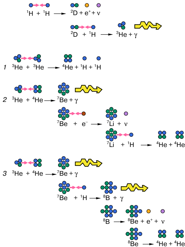
Рис. 1. Протон-протонный цикл.
