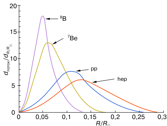
Рис. 4. Доля нейтрино, генерированных на различных расстояниях от центра Солнца, R – расстояние от центра, R_{\odot} – радиус Солнца.
