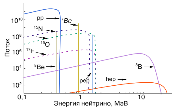
Рис. 3. Энергетический спектр солнечных нейтрино. Для нейтрино с непрерывным энергетическим спектром приведено число нейтрино на 1 \text{ см}^{-2} \cdot \text{с}^{-1} \cdot \text{МэВ}^{-1} на 1 а.е., для монолинии – нейтрино на 1 \text{ см}^{-2} \cdot \text{с}^{-1} .
