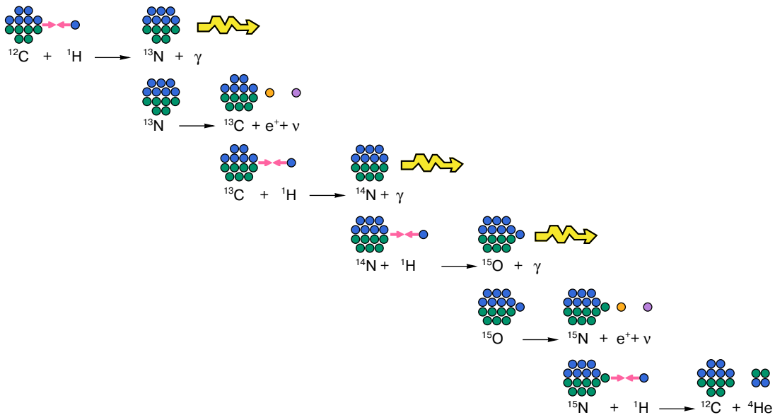
Рис. 2. Углеродно-азотный цикл.
