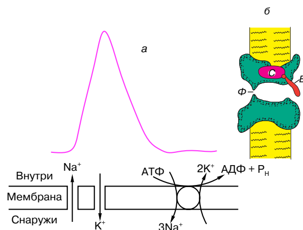
Рис. 2. Схема генерации ПД в нервном волокне: а – пассивные потоки ионов \text{Na} и \text{K} формируют пиковую часть ПД. \text{Na}^+ , \text{K}^+ -АТФаза восстанавливает нарушенное соотношение этих ионов; б – схема строения ионного канала, \Phi – селективный фильтр, B – ворота, C – сенсор, то есть часть канала, чувствительная к напряжению на мембране и связанная с воротами.
