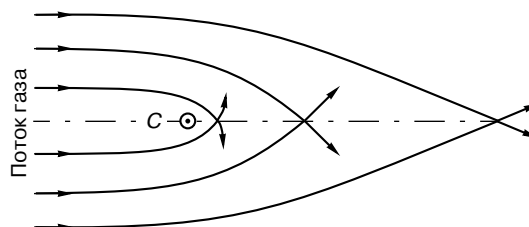
Рис. 2. Фокусировка массивным космическим телом C (Солнцем или звездой) набегающего потока частиц.
