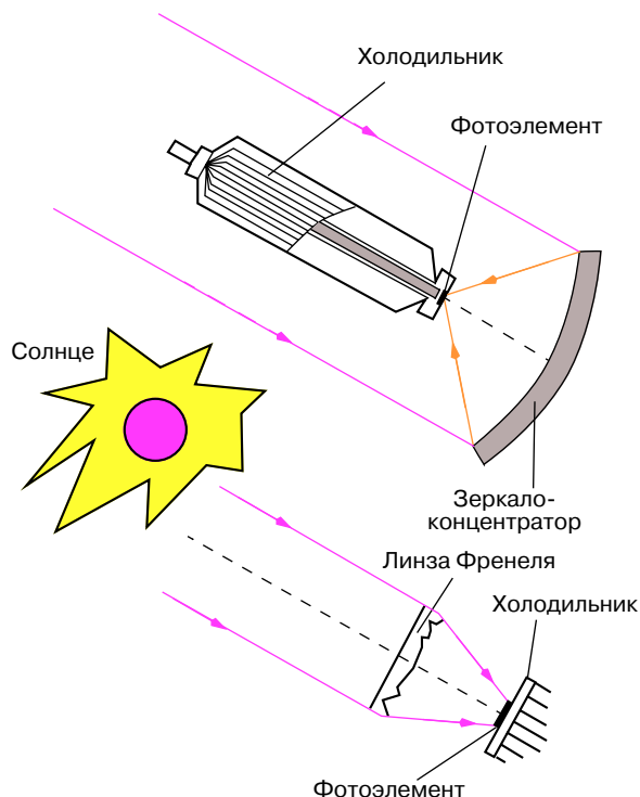
Рис. 3. Схемы фотоэлектрических энергоустановок с концентраторами солнечного излучения.
