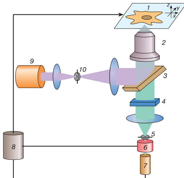
Рис. 3. Упрощенная схема установки для флуоресцентной КЛСМ: 1 — сканируемый в трех направлениях предметный столик, 2 — объектив микроскопа (инвертированный), 3 — дихроичное зеркало, 4 — отсекающий фильтр, 5 — диафрагма детектора, 6 — спектрограф (для выделения нужной полосы флуоресценции), 7 — ФЭУ, 8 — блок регистрации и управления установкой, 9 — лазер, 10 — диафрагма осветителя
