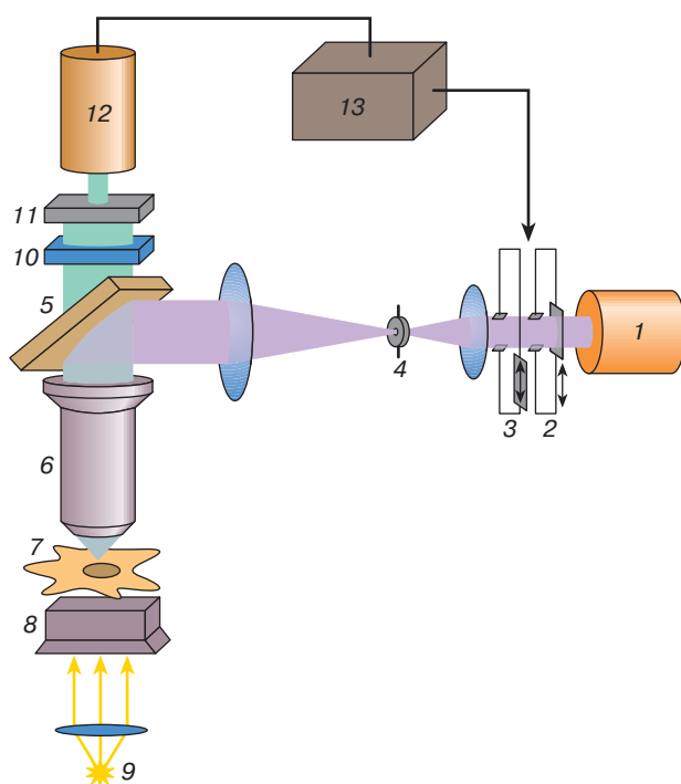
Рис. 1. Упрощенная схема установки для исследования ВФПФ: 1 – лазер, 2 и 3 – аттенюаторы (ослабители луча), 4 – диафрагма, 5 – дихроичное зеркало, отражающее падающий свет и пропускающее свет возбужденной флуоресценции, 6 – объектив микроскопа, 7 – исследуемая клетка, 8 – конденсор микроскопа, 9 – осветитель, 10 – отсекающий светофильтр, 11 – “зонд” – узкая диафрагма, выделяющая флуоресценцию с исследуемого участка, 12 – ФЭУ, 13 – блок регистрации и управления установкой
