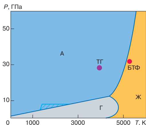
Рис. 4. Фазовая диаграмма углерода. Г – область стабильности графита, А – алмаз, Ж – жидкой фазы углерода. Заштрихована область статического синтеза. Точки – состояния в детонационной волне смеси 50% ТНТ/50% гексогена (ТГ) и БТФ
